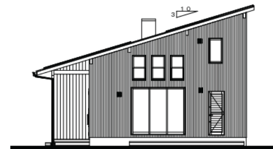
西面立面図 S=1/150
